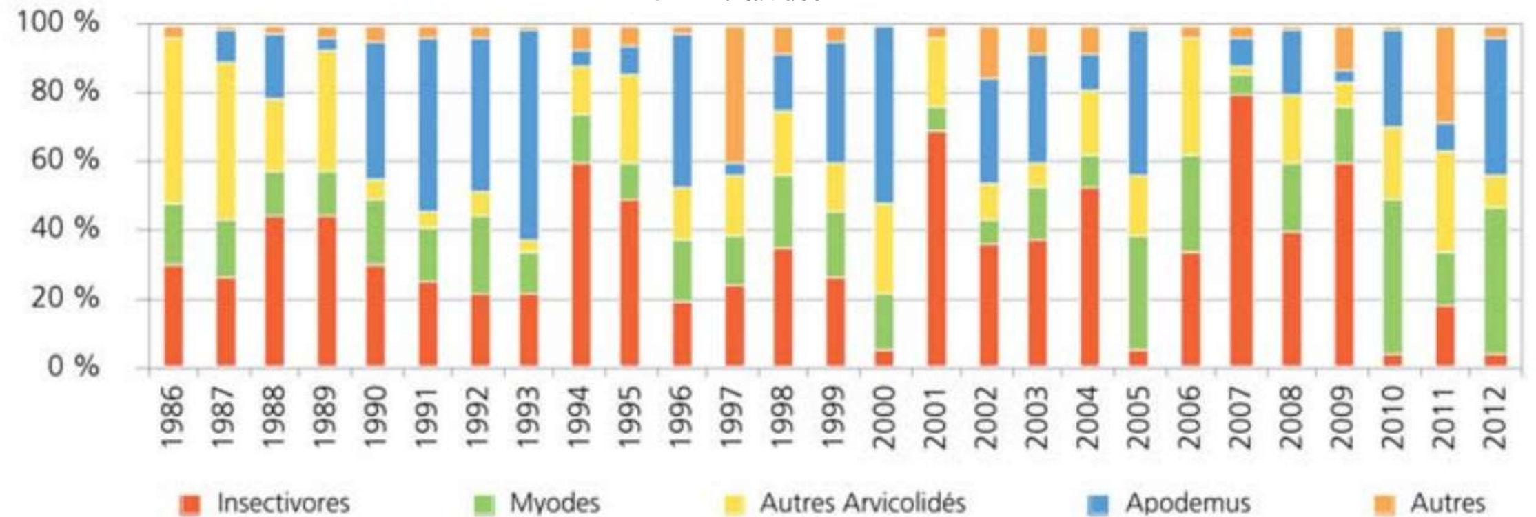
Fig. 10 – Variations annuelles des principaux groupes de proies identifiées dans les fonds de nioirs entre 1986 et 2012. Entre 1986 et 1989, les variations sont faibles et ce sont les campagnols des genres Microtus (Autres Arvicolidés) qui dominant. De 1990 à 1993, les variations annuelles restent faibles, mais ce sont alors les mulots Apodemus qui sont prépondérants. Depuis 1993, les mulots fluctuent de manière plutôt cyclique, avec des pics tous les 3 à 5 ans. Les Insectivores (essentiellement Sorex araneus ) sont des proies de remplacement. Elles sont abondantes dans les fonds de nioirs lors des « mauvaises années », en particulier entre 2001 et 2004, et surtout en 2007 et 2009.
